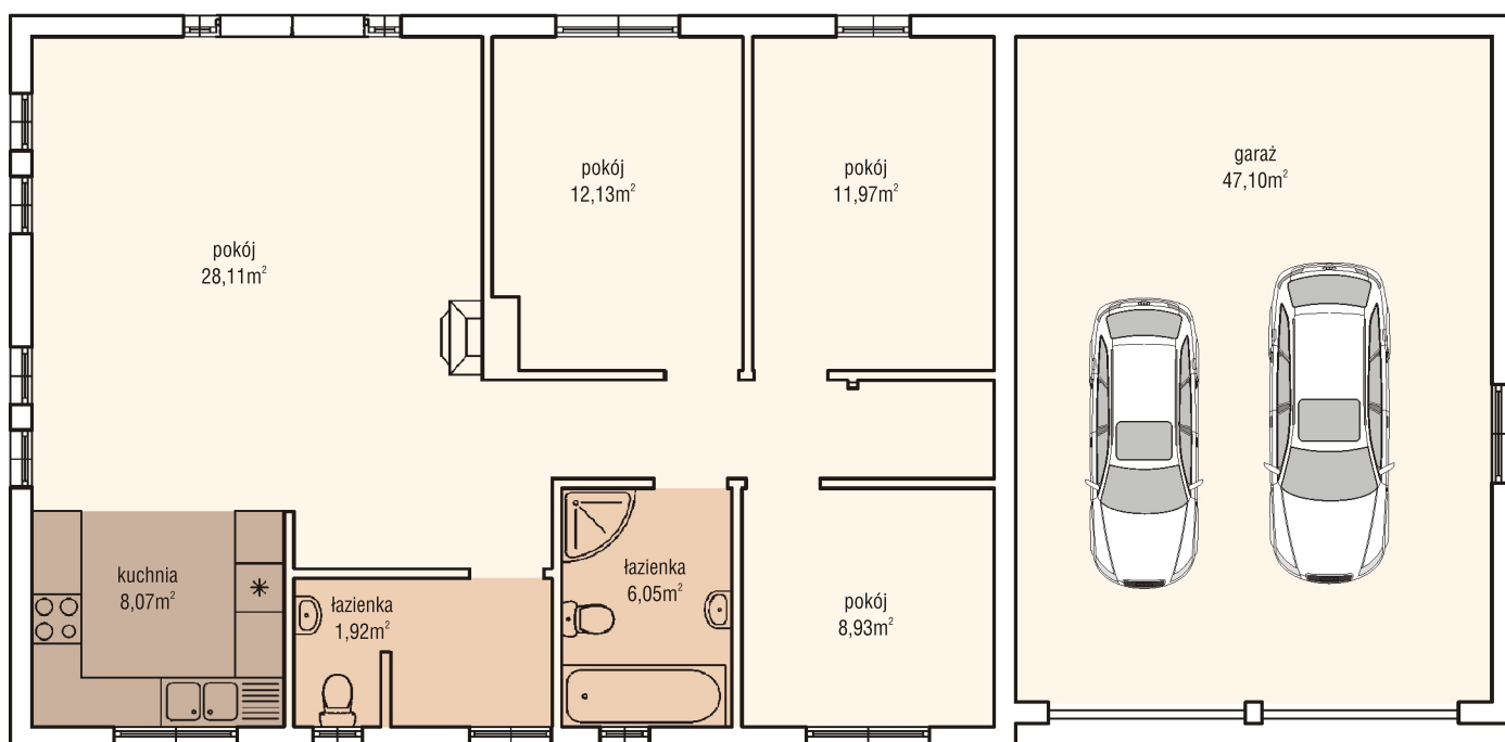
rzut parteru
