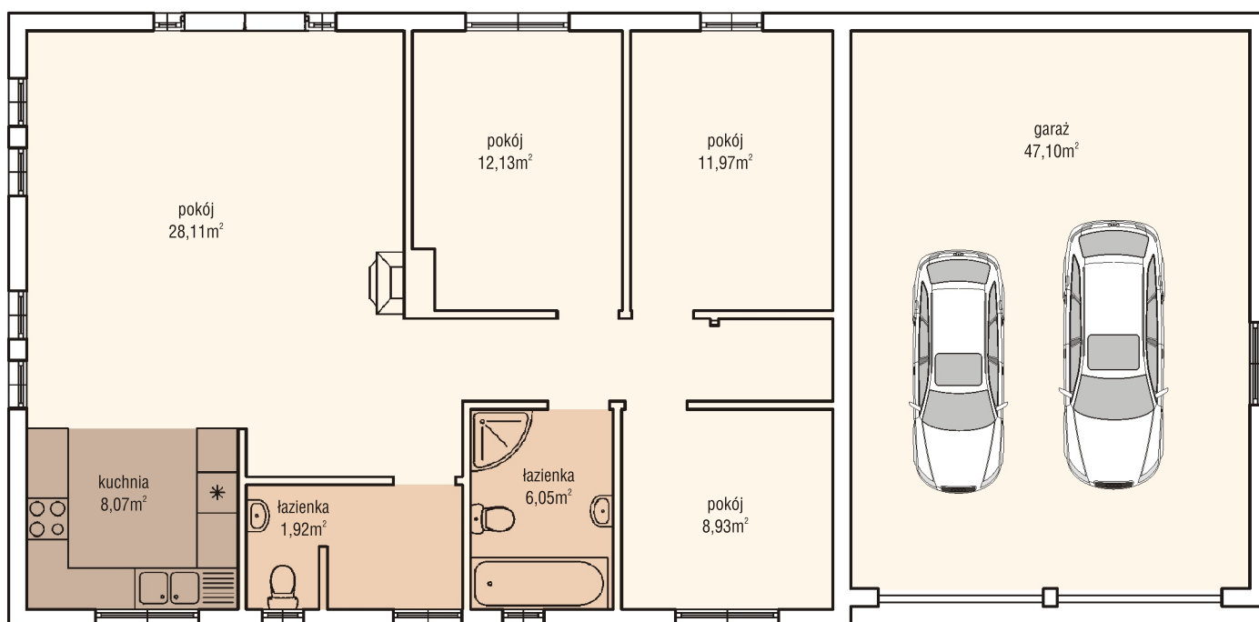
rzut parteru
