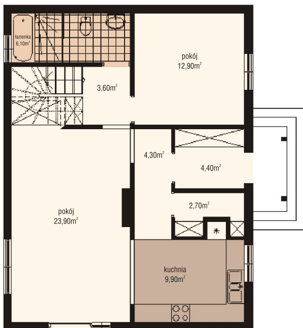
rzut parteru
